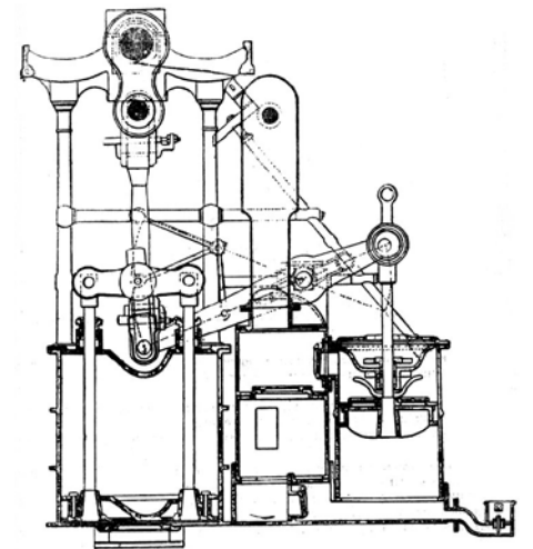
Паровая машина с кривошипно-шатунным механизмом для военного парохода «Геркулес»
